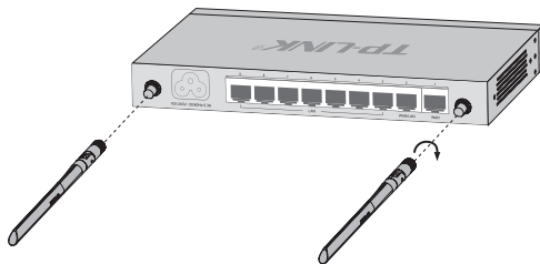
图2-2 安装天线示意图
