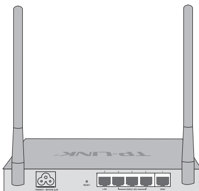
图1-2 TL-WAR302后面板示意图
